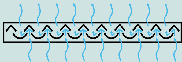
Schéma en coupe d'un filtre No-Drop à lames entrecroisées.
