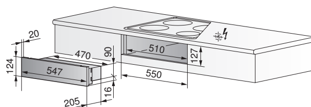
SIBIR | Réchaud ER 4
