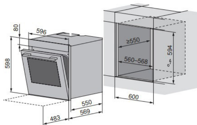
Four à encastrer norme EURO SIBIR | EB Tritherm V600
