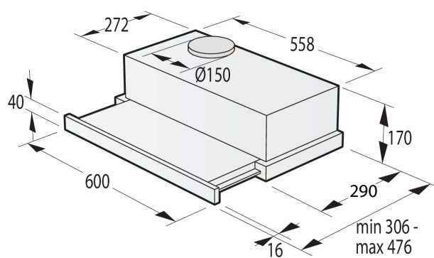
Gorenje | TH62E4X (Gorenje)
