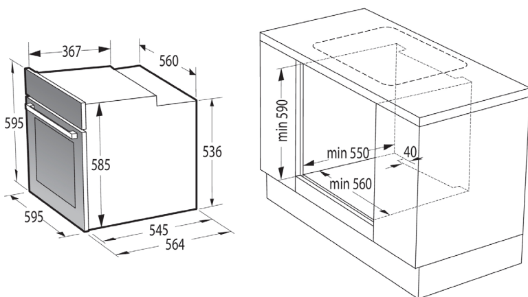
Cuisinières à encastrer norme EURO Gorenje | BCS6737E06X / BC6737E02X
