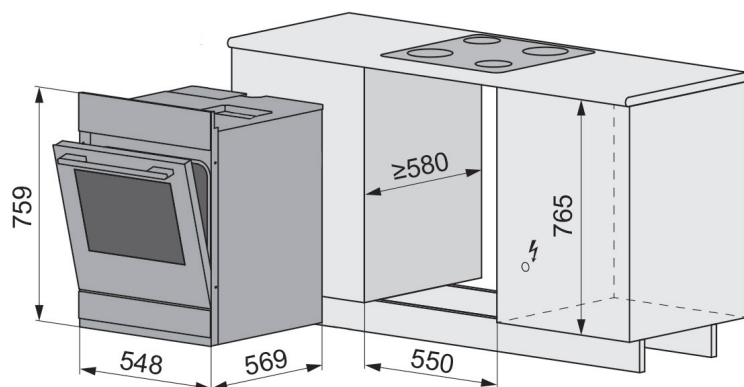
Cuisinières à encastrer norme SMS SIBIR | EH Tritherm 4 V200 / V400 / V600
