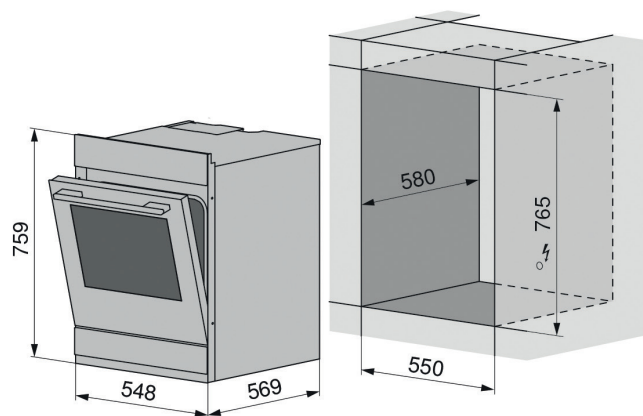
Four à encastrer norme SMS SIBIR | EB Tritherm V400 / V600
