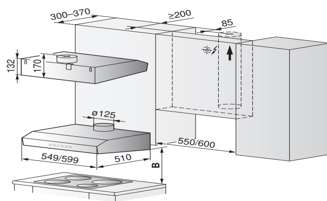
SIBIR | DFNA55 + DFNA60
