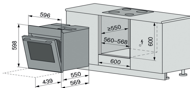
Cuisinières à encastrer norme EURO SIBIR | EH Tritherm V600 / Tritherm 4 V400
