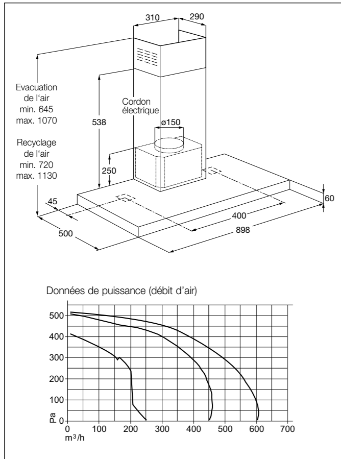
Hotte design murale AWH9416AM (jusqu'en août 2024)
