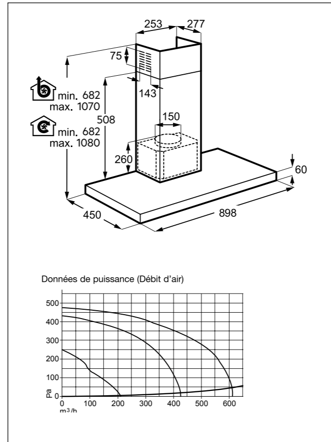
Hotte design murale AWH9416AM (à partir d'août 2024)
